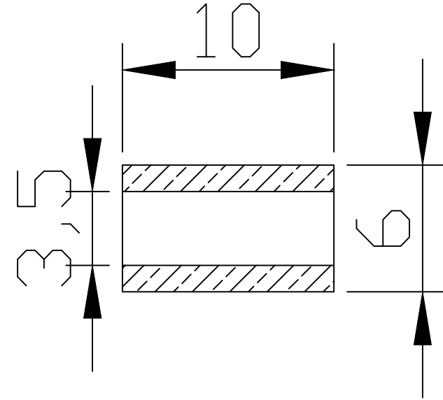
Sezione A-A
