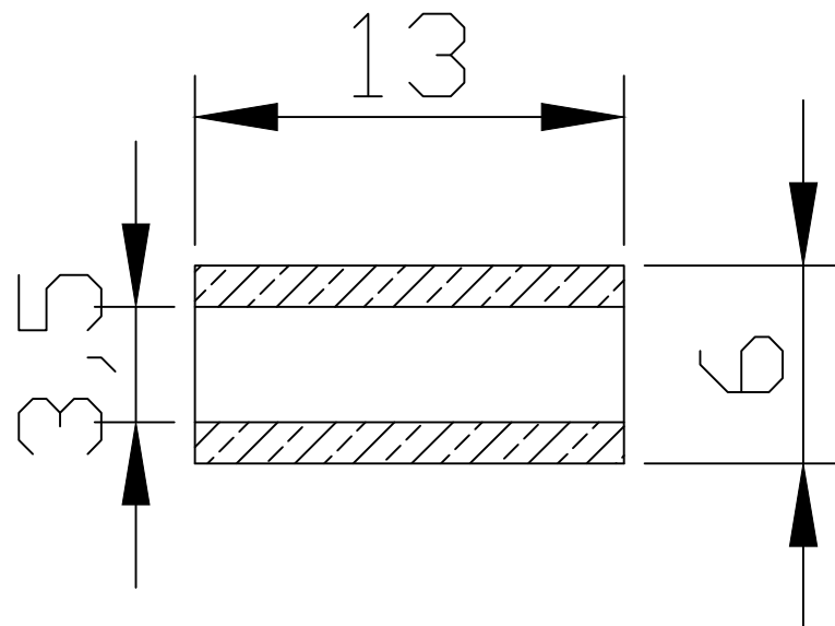
Sezione A-A
