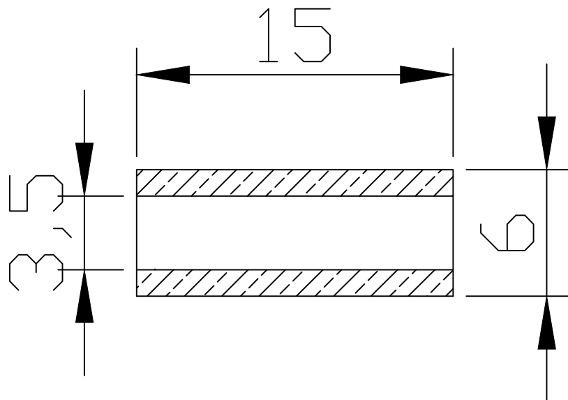
Sezione A-A
