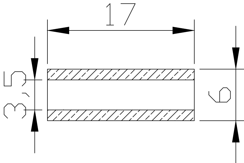
Sezione A-A
