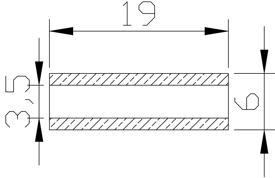
Sezione A-A
