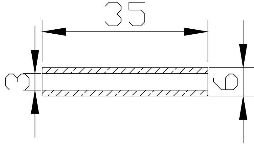
Sezione A-A
