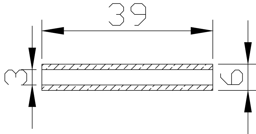
Sezione A-A
