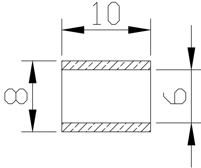
Sezione A-A
