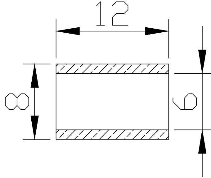
Sezione A-A
