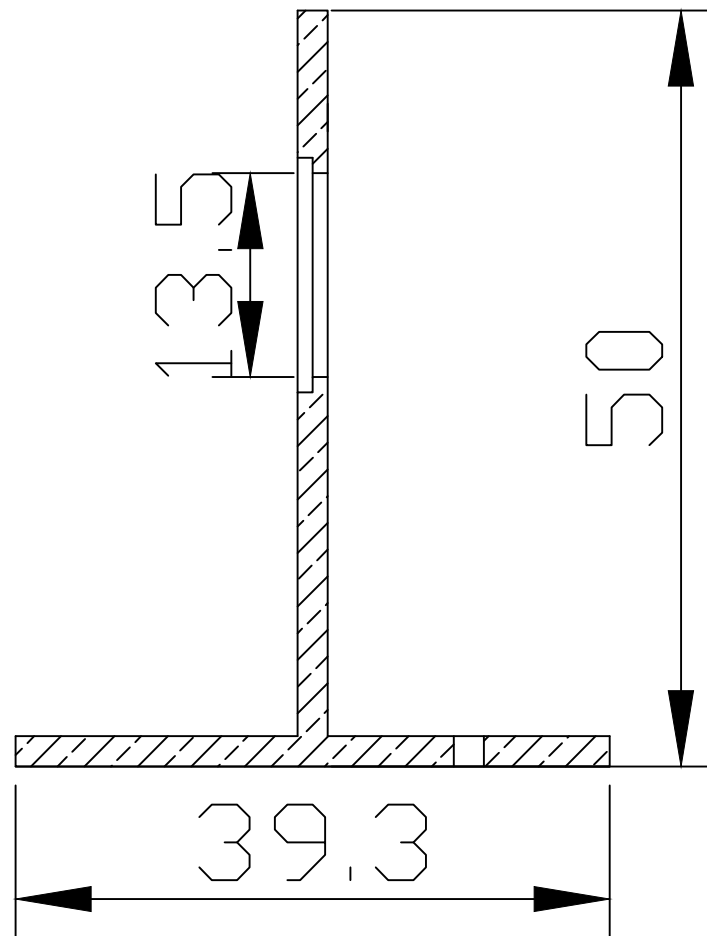
Sezione A-A
